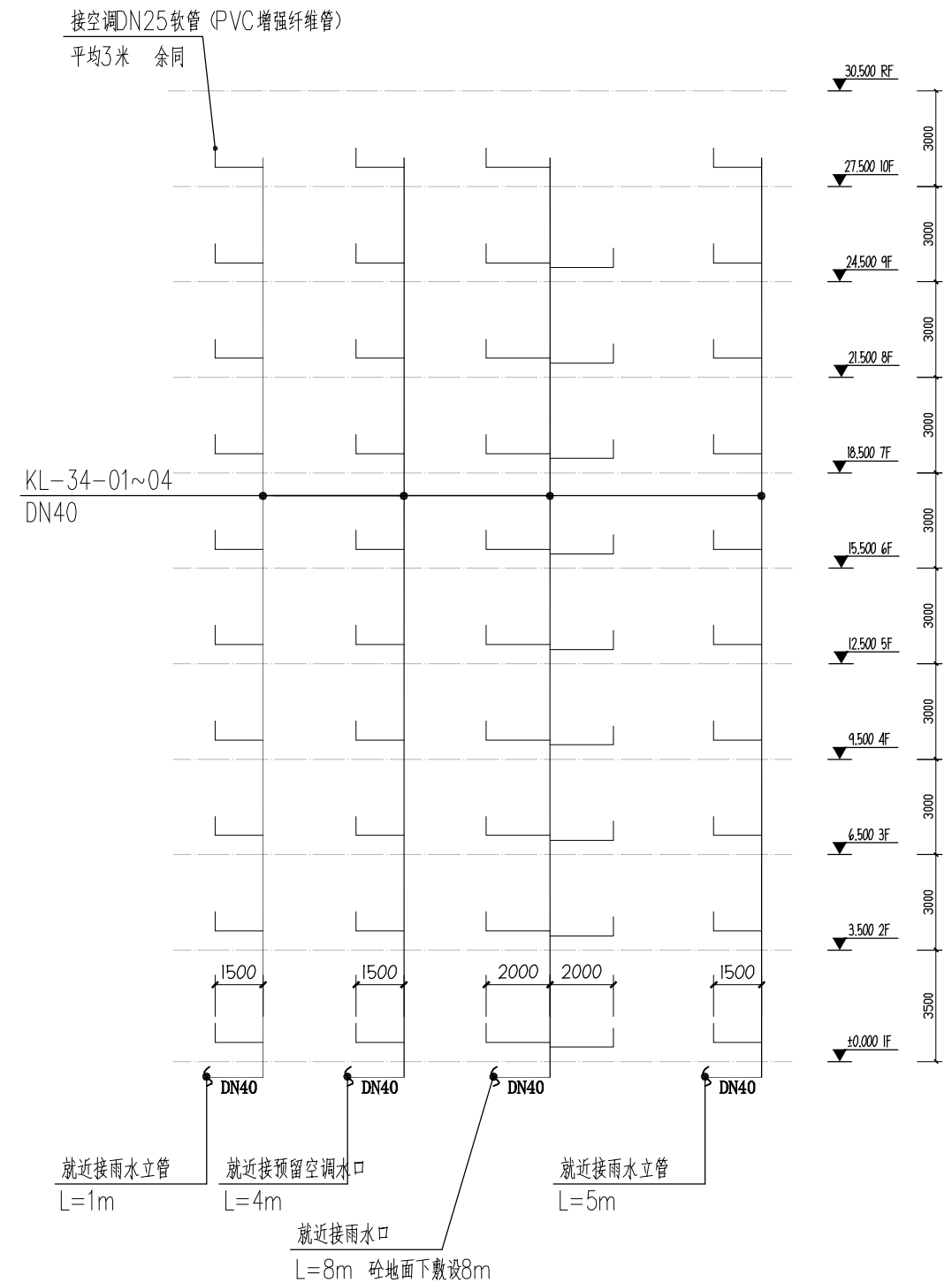
34栋空调排水管立面图 1:200
