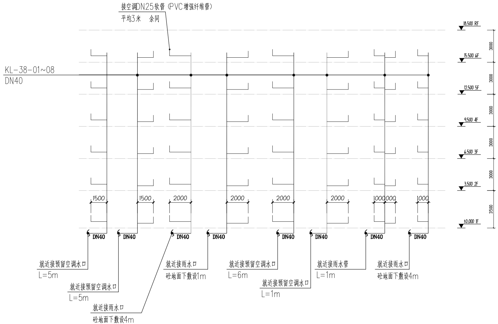
38栋空调排水管立面图 1:200
