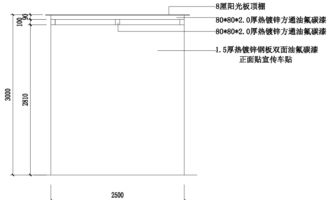
侧立面图 尺寸根据平面图调整
