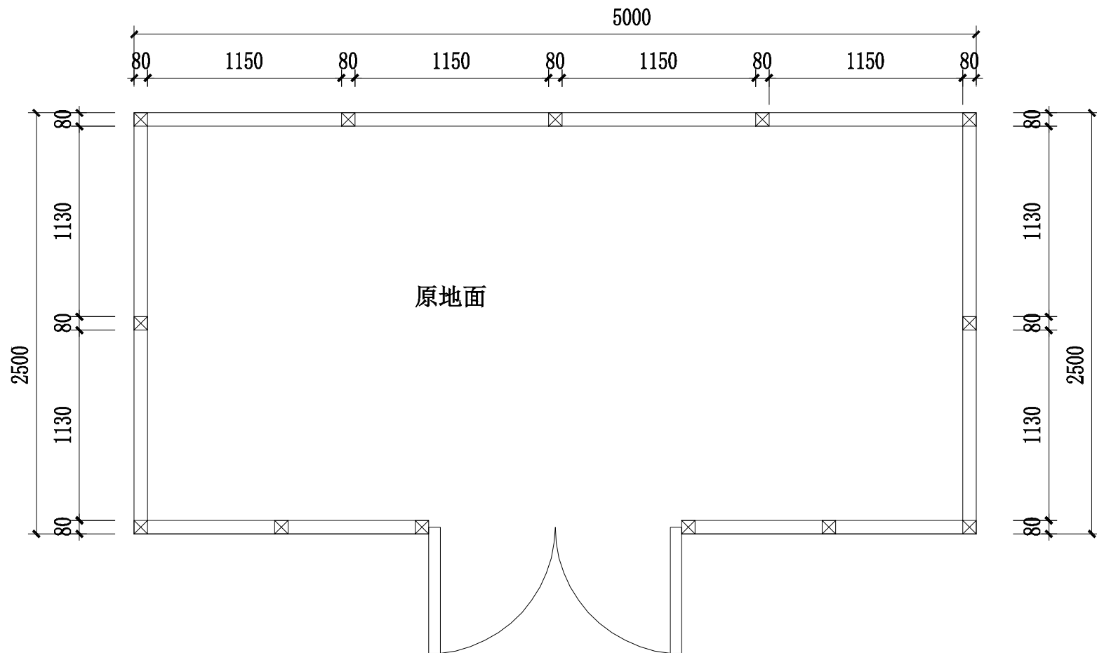
凯丰花园 平面布置图
