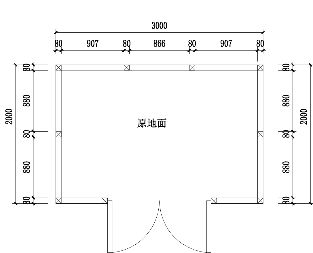
辉煌时代大厦 平面布置图
