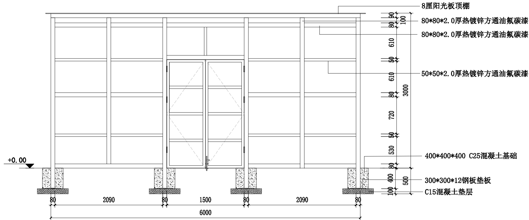
正面钢骨架立面图 尺寸根据平面图调整
