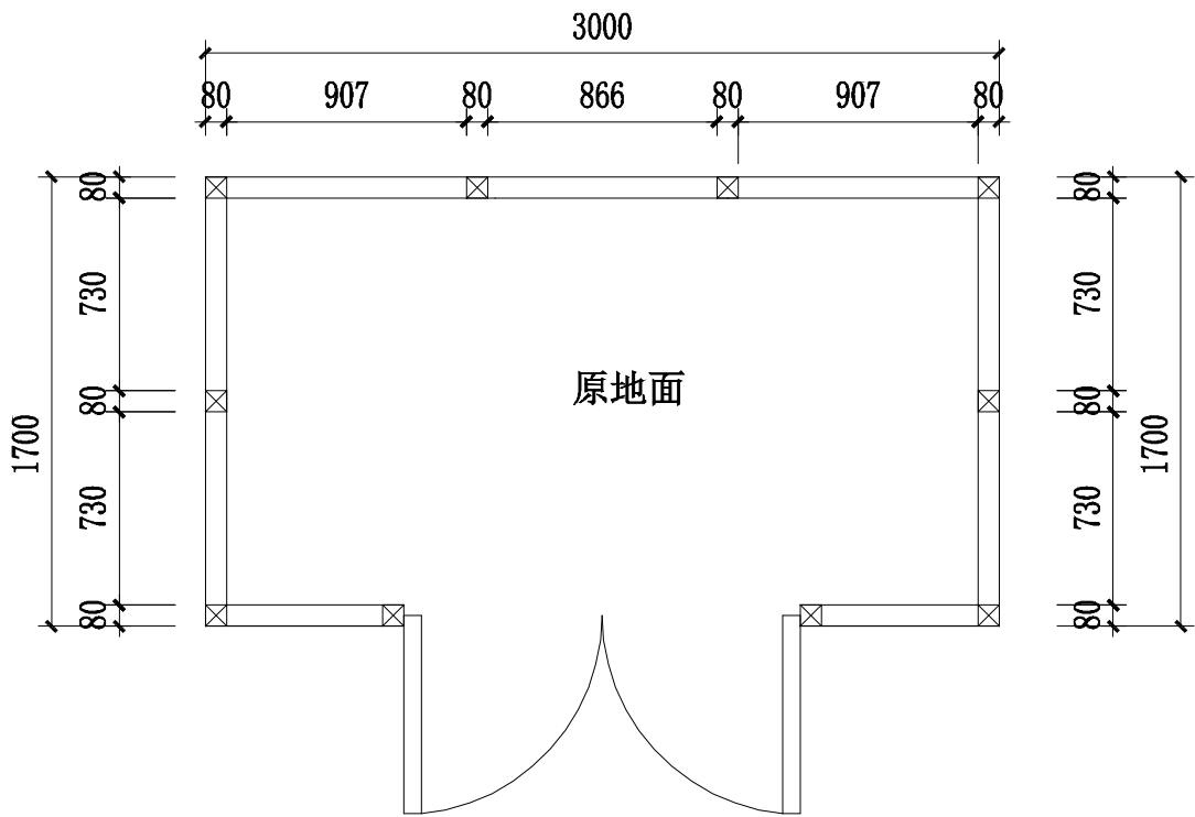
福丰楼 平面布置图
