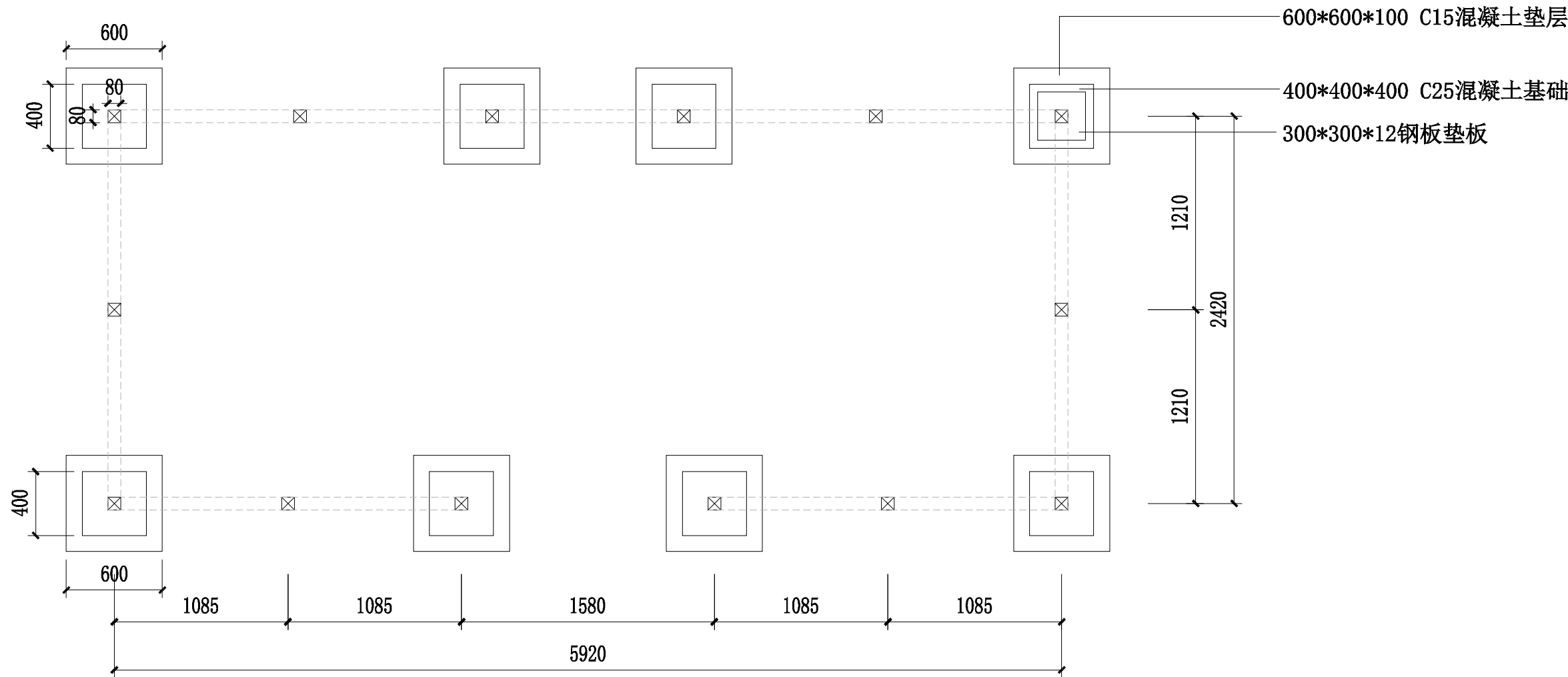
标准地面基础布置图 尺寸根据平面图调整
