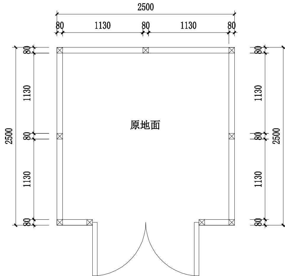
合旺阁 平面布置图
