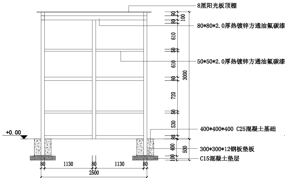
侧面钢骨架立面图 尺寸根据平面图调整
