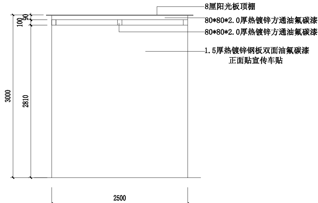
侧立面图2 尺寸根据平面图调整
