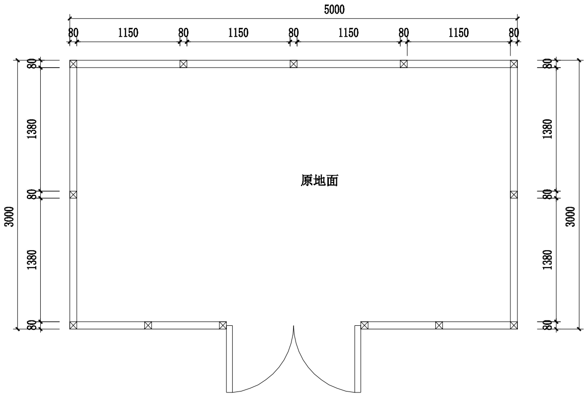
公安街3号 平面布置图
