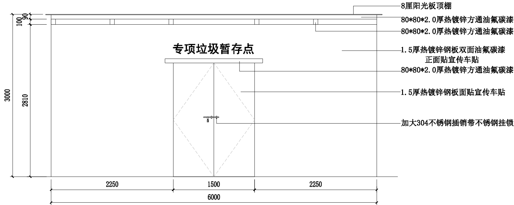
正立面图 尺寸根据平面图调整
